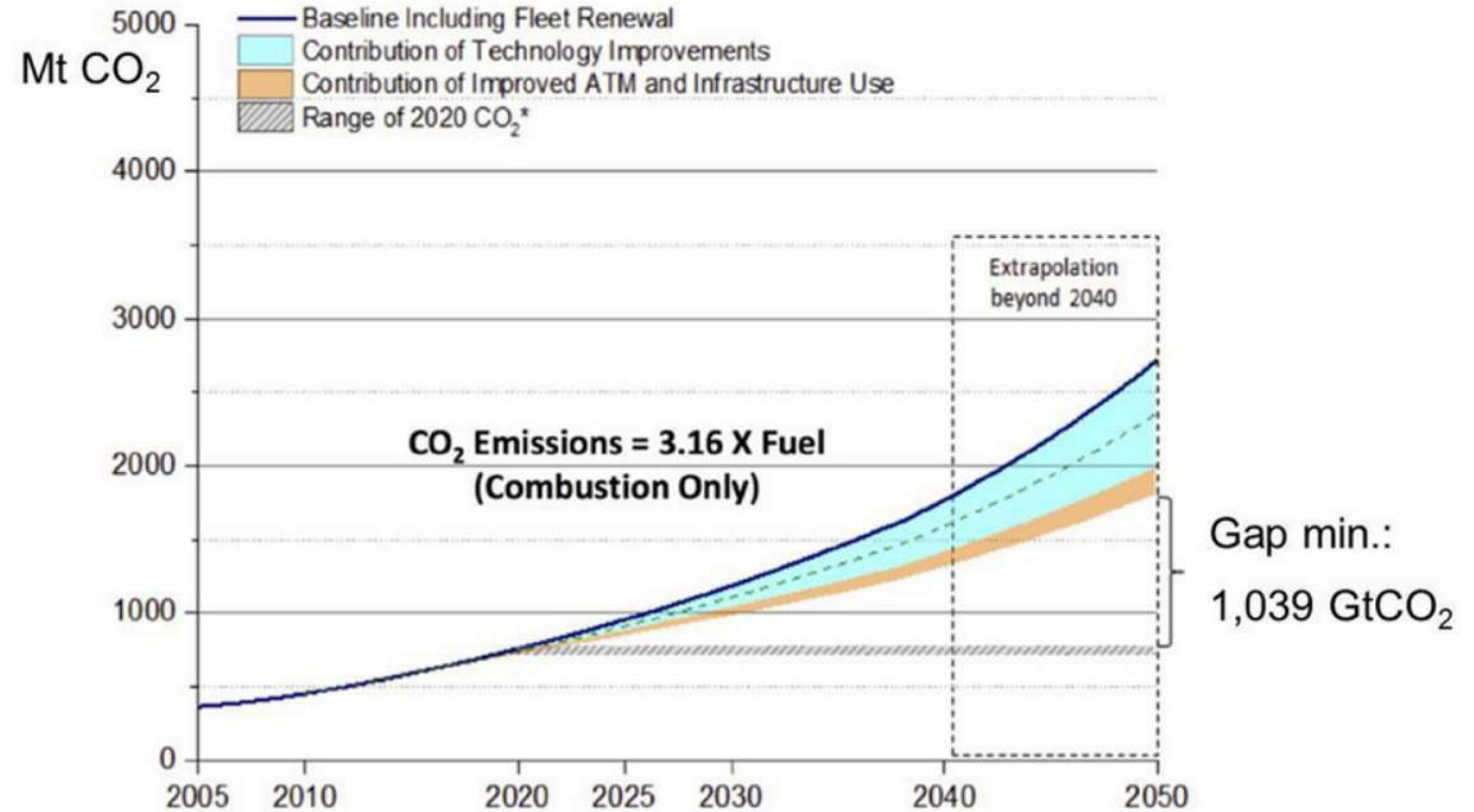
Figure 3 : émissions de CO 2 de l'aviation civile internationale – projections à 2050 (source : ICAO, 2015)
